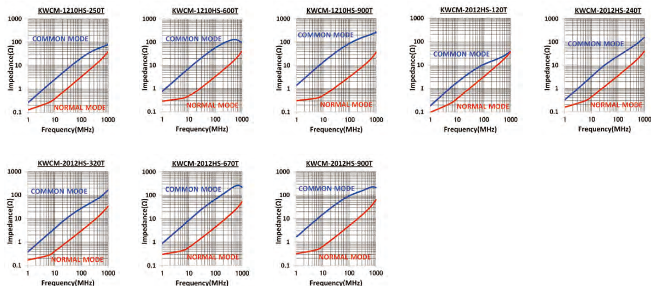
インピーダンス周波数特性 Impedance vs frequency
