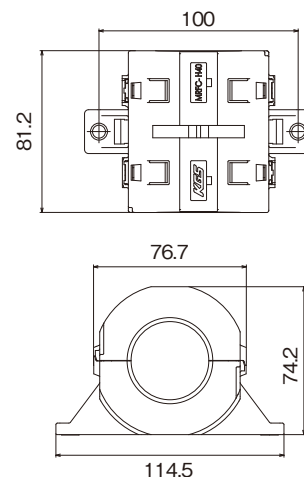
上下パーツ嵌合前状態 Split parts of top and bottom before assembly
