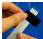
③ケーブルを挟みこむようにA部とB部を貼り合わせます
