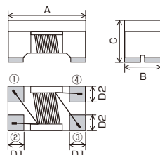
■ 外形寸法 Outside dimensions
