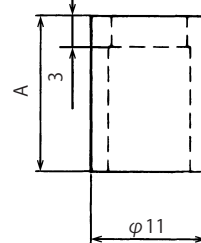
3mmねじ用カラー Collar for 3mm screw
