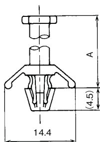
KGPS-S・KGSP-M
