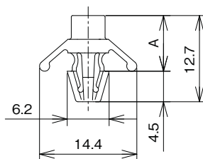
KGPS-3.5S-N
