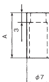
3mmねじ用カラー Collar for 3mm screw
