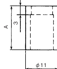
4mmねじ用カラー Collar for 4mm screw
