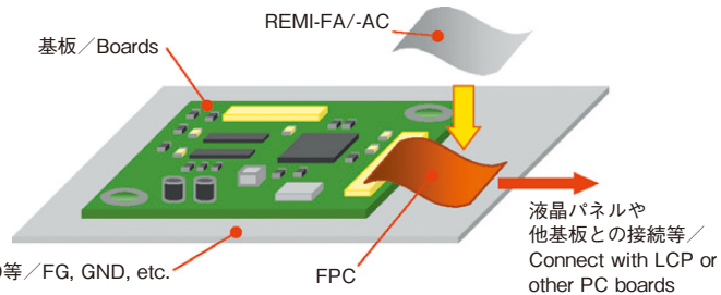
例) FPCをシールドしてFGにグランディング Application example) Shielding and frame-grounding for FPC
