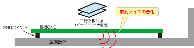
2つの金属間の共振構造は、平行平板共振構造
