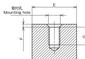
止まり穴 Blind Hole
